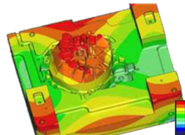
DIE STRESS ANALYSIS
