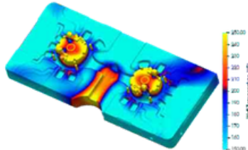
THERMAL DIE ANALYSIS
